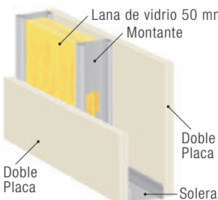
Tabique doble con lana de vidrio
