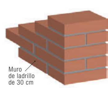
Muro de ladrillo común de 30 cm
