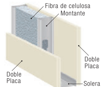
Tabique doble con celulosa
